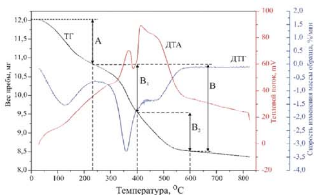
Дериватограмма ископаемого микрофрагмента челюсти водяной полевки ( Arvicola terrestris ) из Четвертичных отложений Урала
