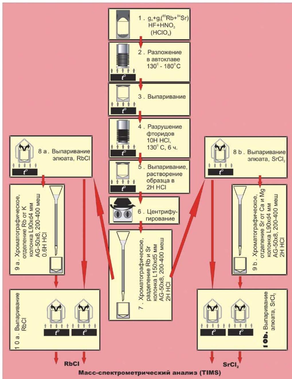
Схема пробоподготовки геологического материала для анализа изотопного состава Rb и Sr масс-спектрометрическим методом изотопного разбавления (ID).
