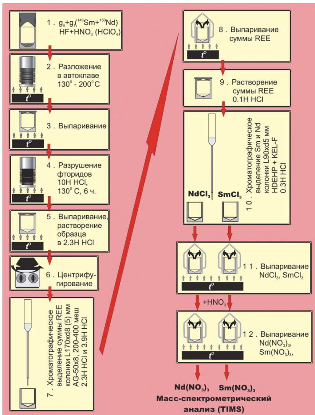
Схема пробоподготовки геологического материала для анализа изотопного состава Sm и Nd масс-спектрометрическим методом изотопного разбавления (ID).
