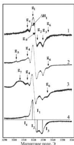
ЭПР спектры зубной эмали человека
