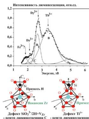
Спектр люминесценции минерала циркона и структурные модели центров
