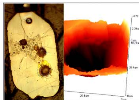
Микрозерно циркона после лазерной абляции (данные ACM)
